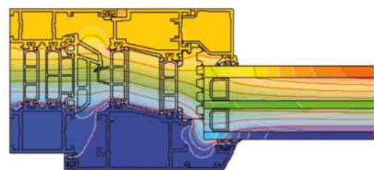
przykładowy rozkład izoterm dla złożenia ościeżnicy i skrzydła okiennego systemu SP OUT i+ (SP 010 + SP 521)
