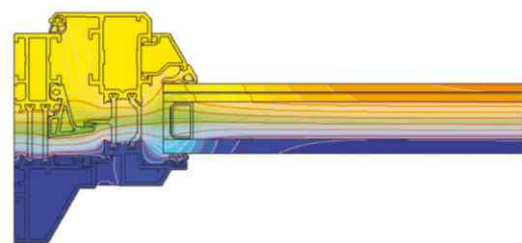
przykładowy rozkład izoterm dla złożeń ościeżnicy i skrzydła okiennego systemu ST1000 (ST1010 + ST1020)
